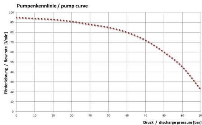
Caudal (l/min) / Presión (Bar)
